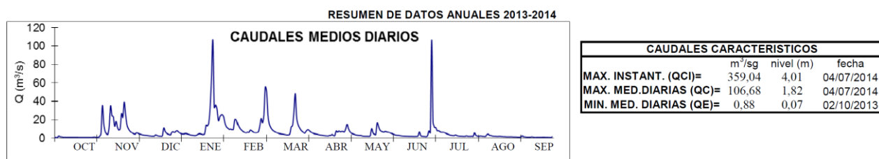
Figura 4 Caudales medios diarios y caudales característicos ( \text{m}^3/\text{s} ) de la estación de Oharriz (río Baztan).
