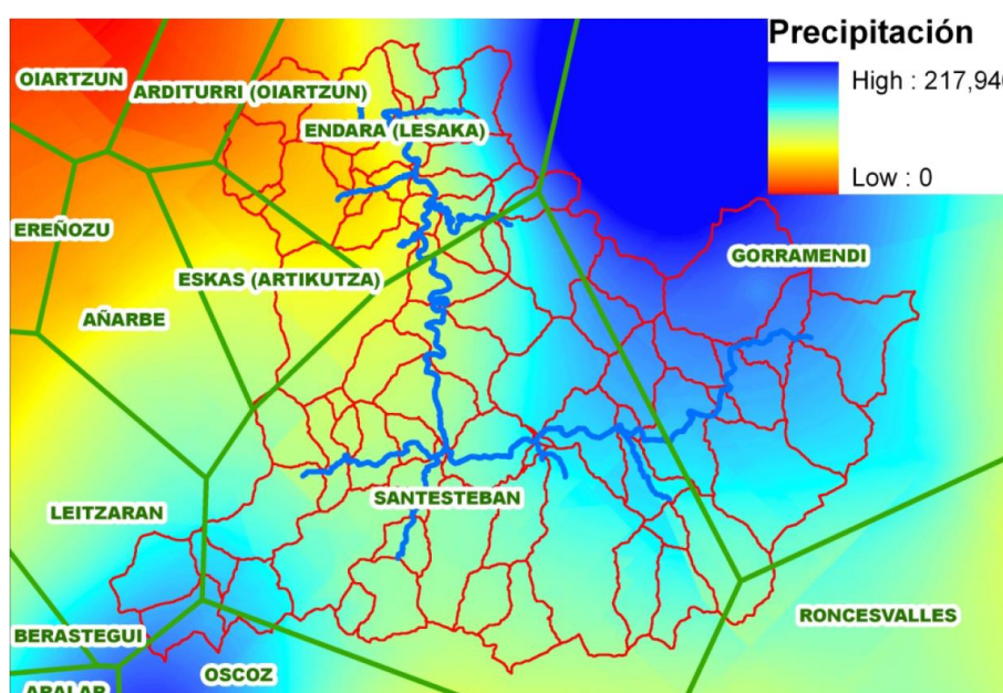
Figura 3 Precipitación total acumulada (mm) del evento del 04/05/2007 en la cuenca del Bidasoa.
