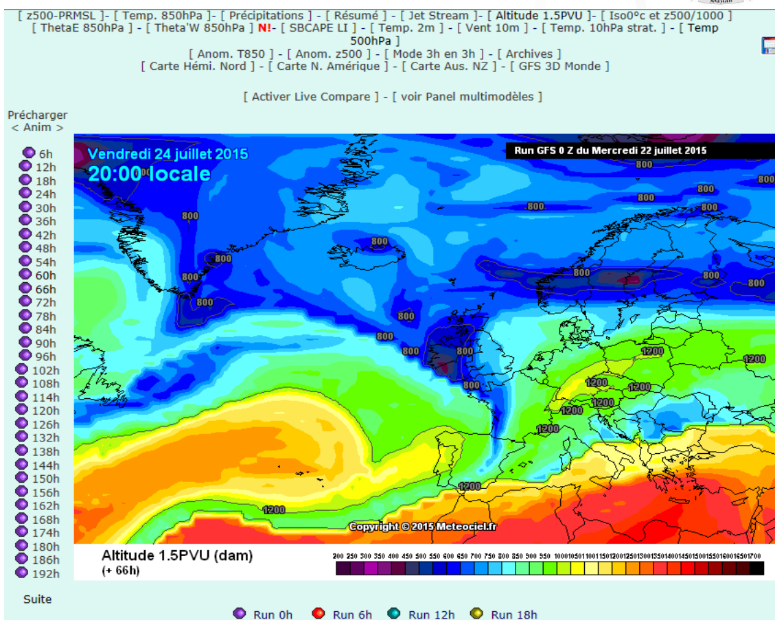
Figura 35 Imagen de la altura geopotencial a 1.5 UPV del modelo meteorológico GFS. Los tonos azules permiten identificar estos hundimientos de la tropopausa característicos de una DANA.
