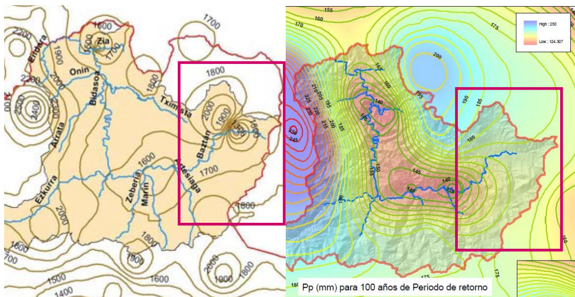
Figura 9 Para toda la cuenca del Bidasoa, enmarcando el rectángulo rosa al valle de Baztan: Precipitaciones promedio anuales (izda.) y precipitaciones máximas en 24 horas (dcha.).
