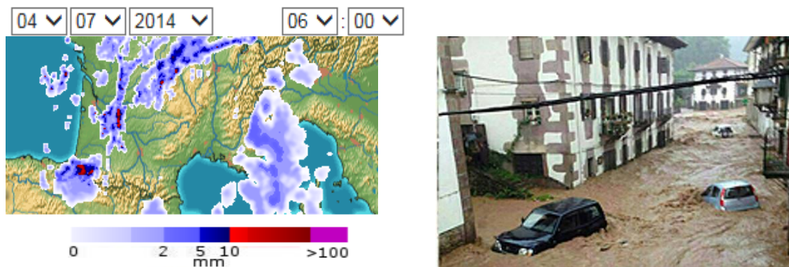
Figura 6 Imagen radar que muestra la distribución espacial de la Precipitación (mm) el 04/07/2014 a las 6:00 (izda.) y fotografía la mañana del mismo día en Elizondo (dcha.).
