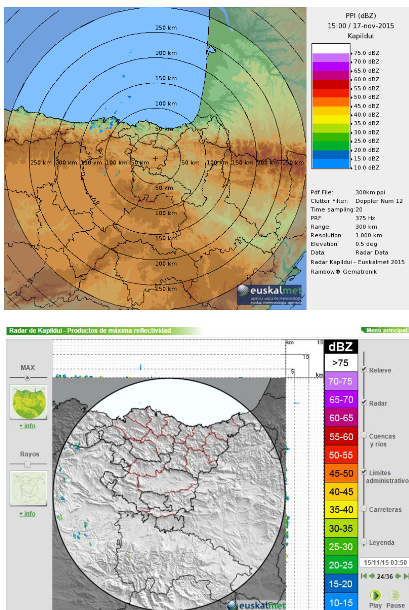
Figura 33 Animación de radar de Kapildui cada 10 minutos en un radio de 100 km (Euskalmet).
